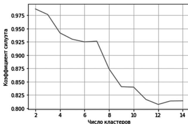
Рис. 1. Зависимость коэффициента силуэта от количества кластеров
